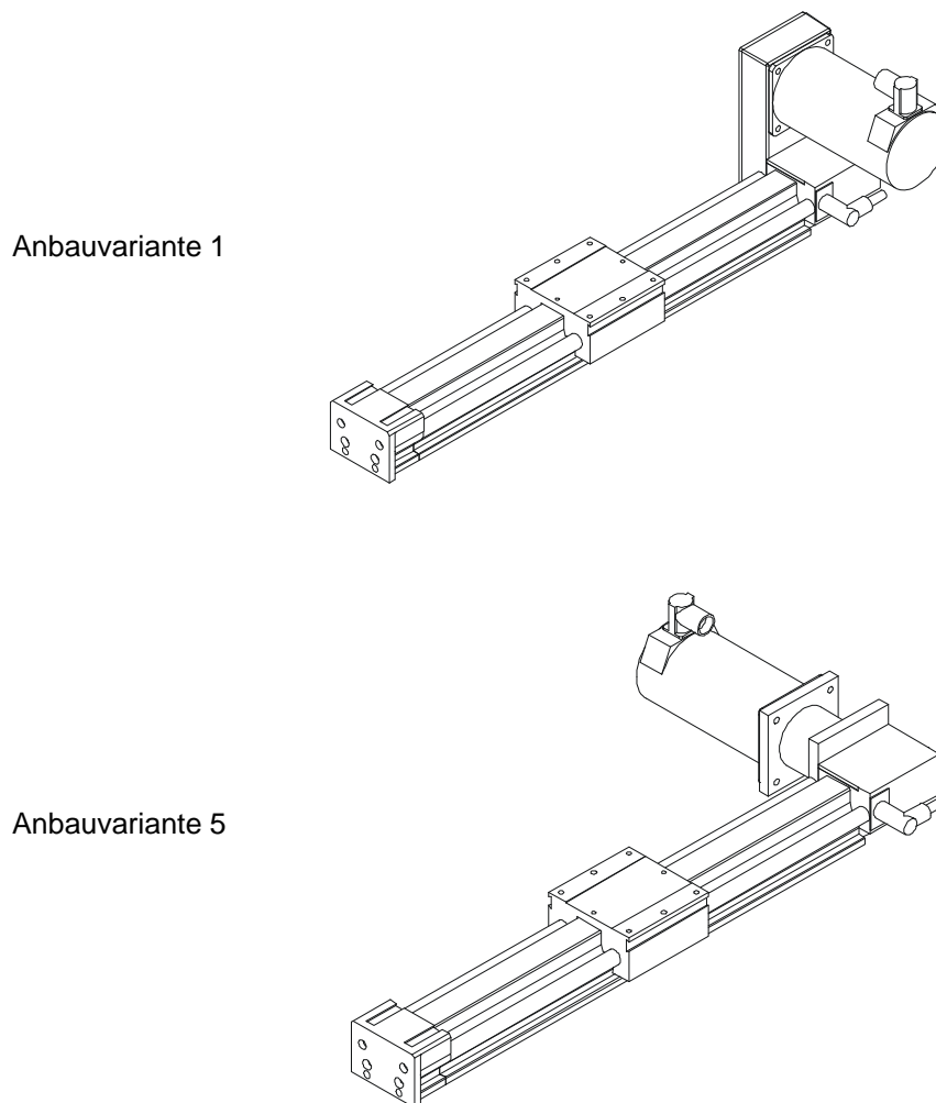
Abbildung 2: Anbauvarianten modul easyLINE
