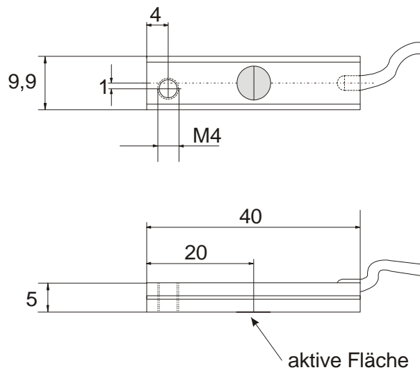
Abbildung 15: Maßskizze Initiator
