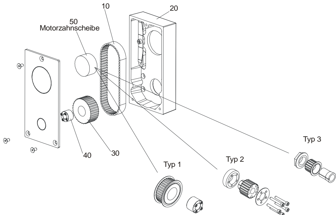
Abbildung 24: easyLINE Riemengetriebe
