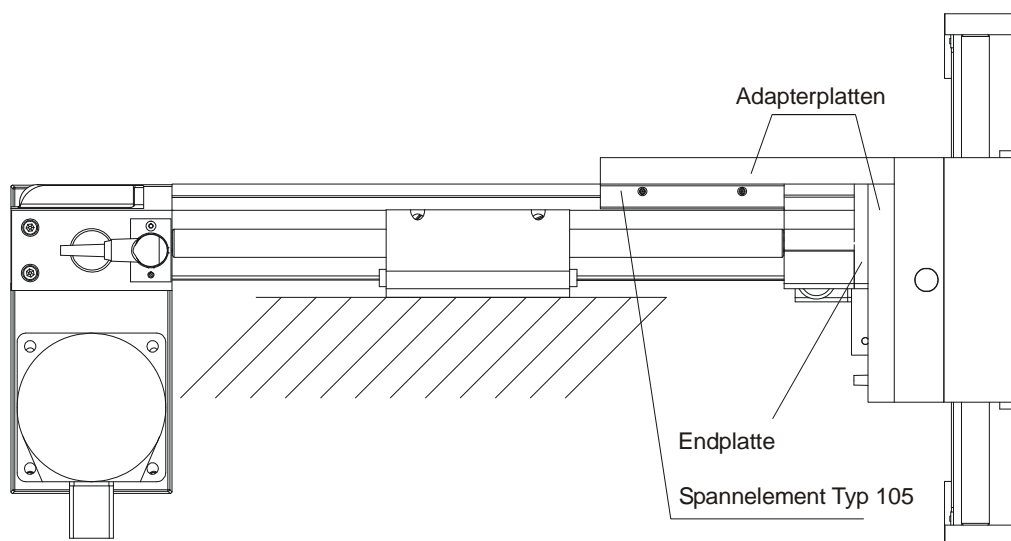
Abbildung 12: Anbaubeispiel
