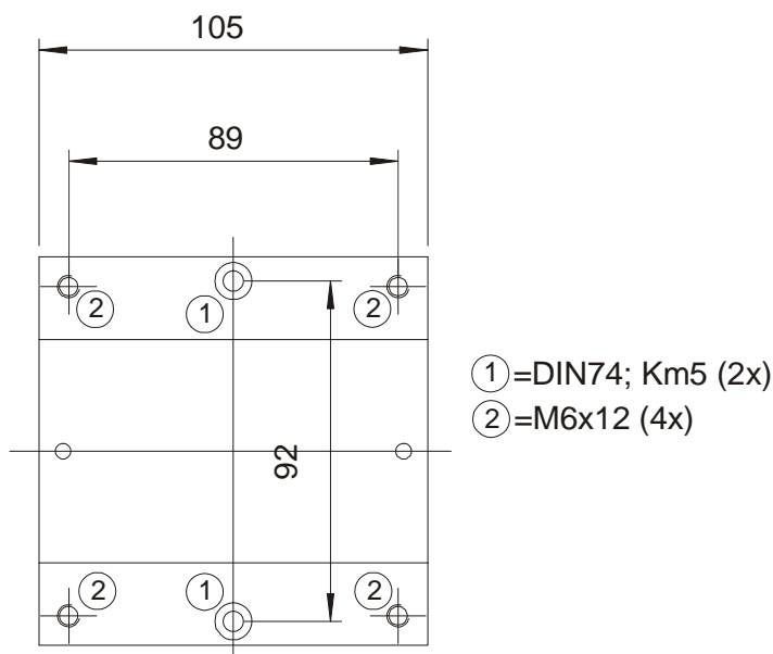
Abbildung 10: Bohrbild Standardschlitten
