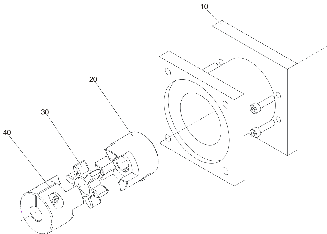
Abbildung 25: easyLINE Flansch i = 1:1
